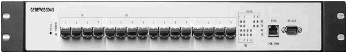
图 2-2 FS3116 千兆设备正面结构
