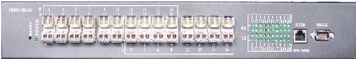
图 2-3 FS3128 千兆设备正面结构
